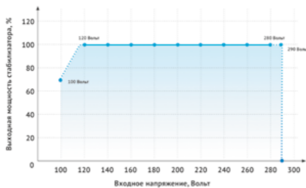
График зависимости мощности от входного напряжения
